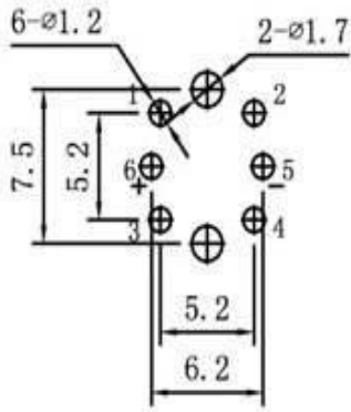
P. C. B. Land Pattern
